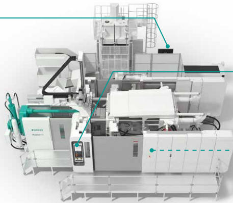
SmartCMS Bildschirm zur Steuerung, Ansicht und Programmierung Ihrer gesamten Zelle.
